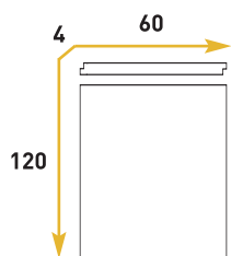
PANNELLO CAPPOTTO
